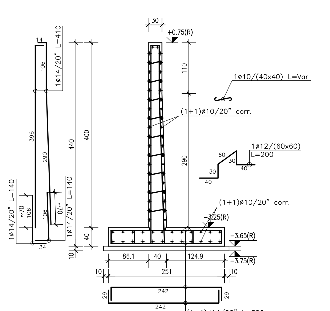
SEZIONE 3-3
