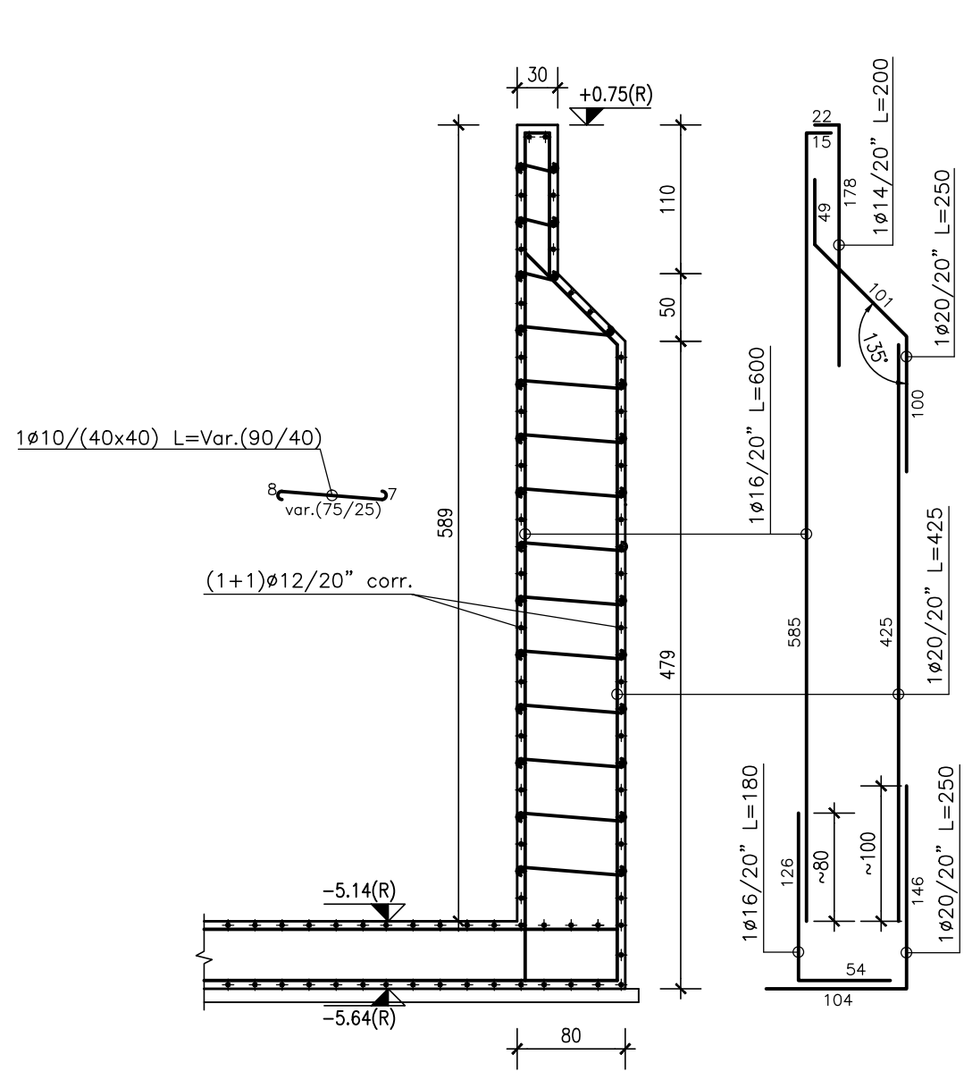
SEZIONE A-A
