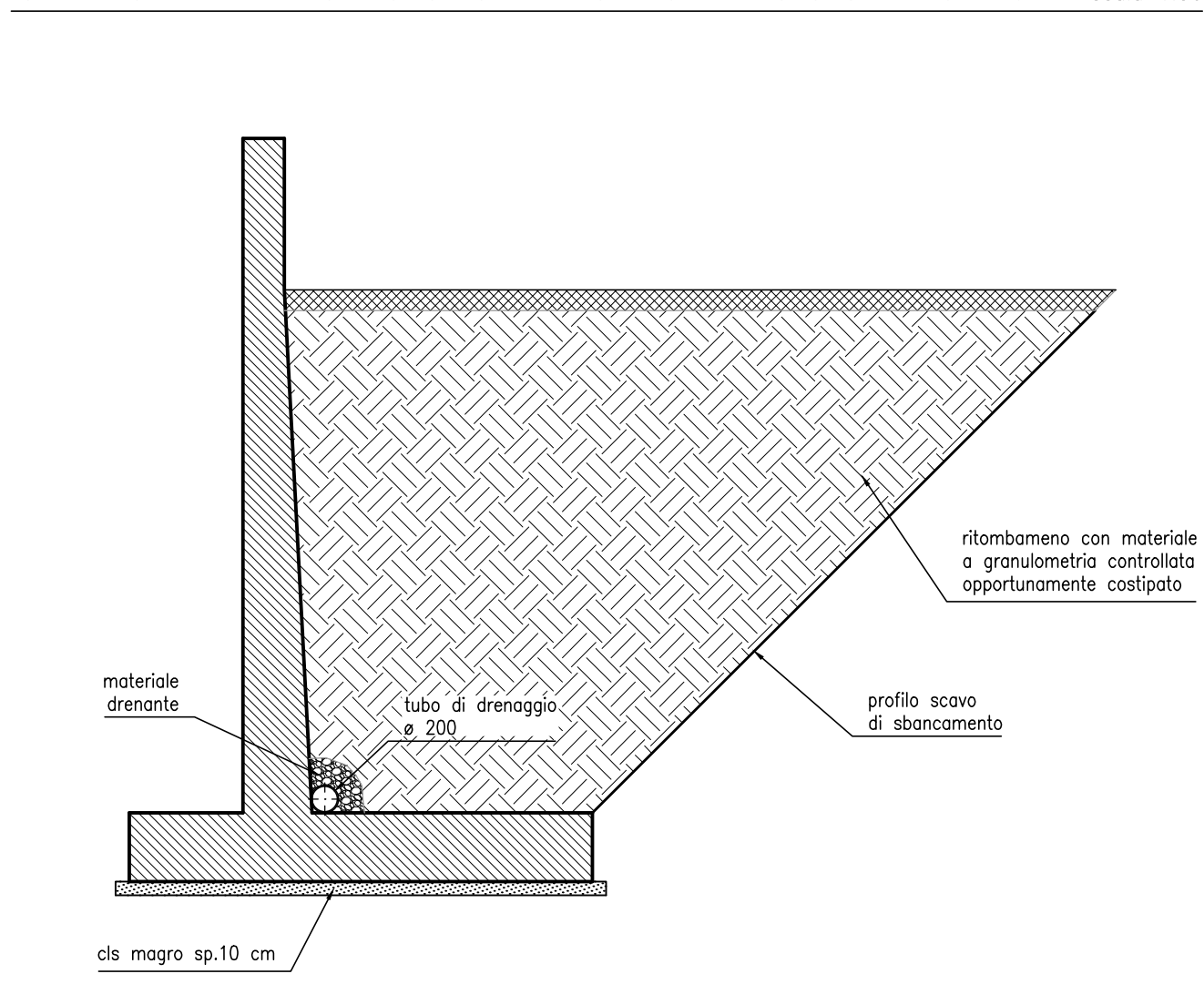
SEZIONE TIPOLOGICA MURO DI SOSTEGNO
