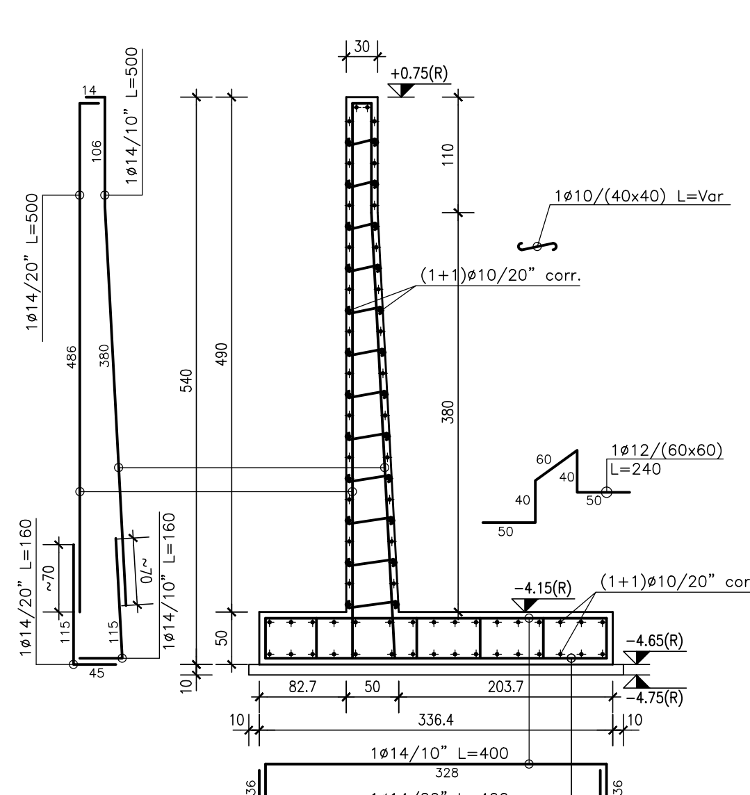
SEZIONE 2-2
