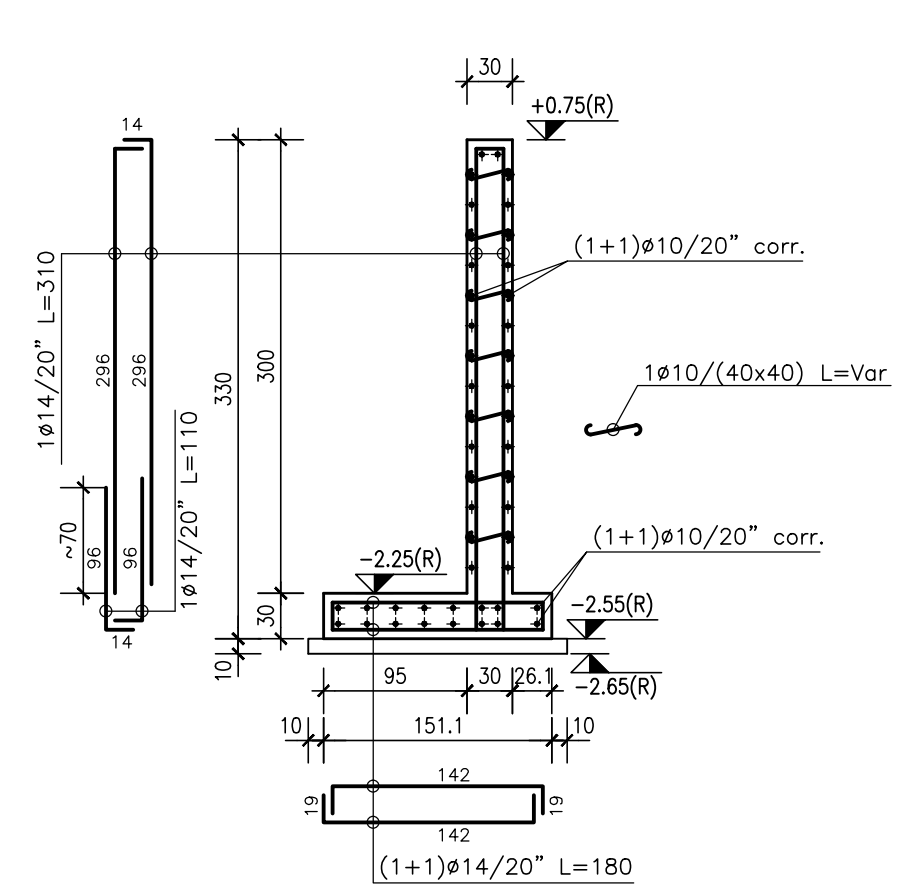
SEZIONE 4-4
