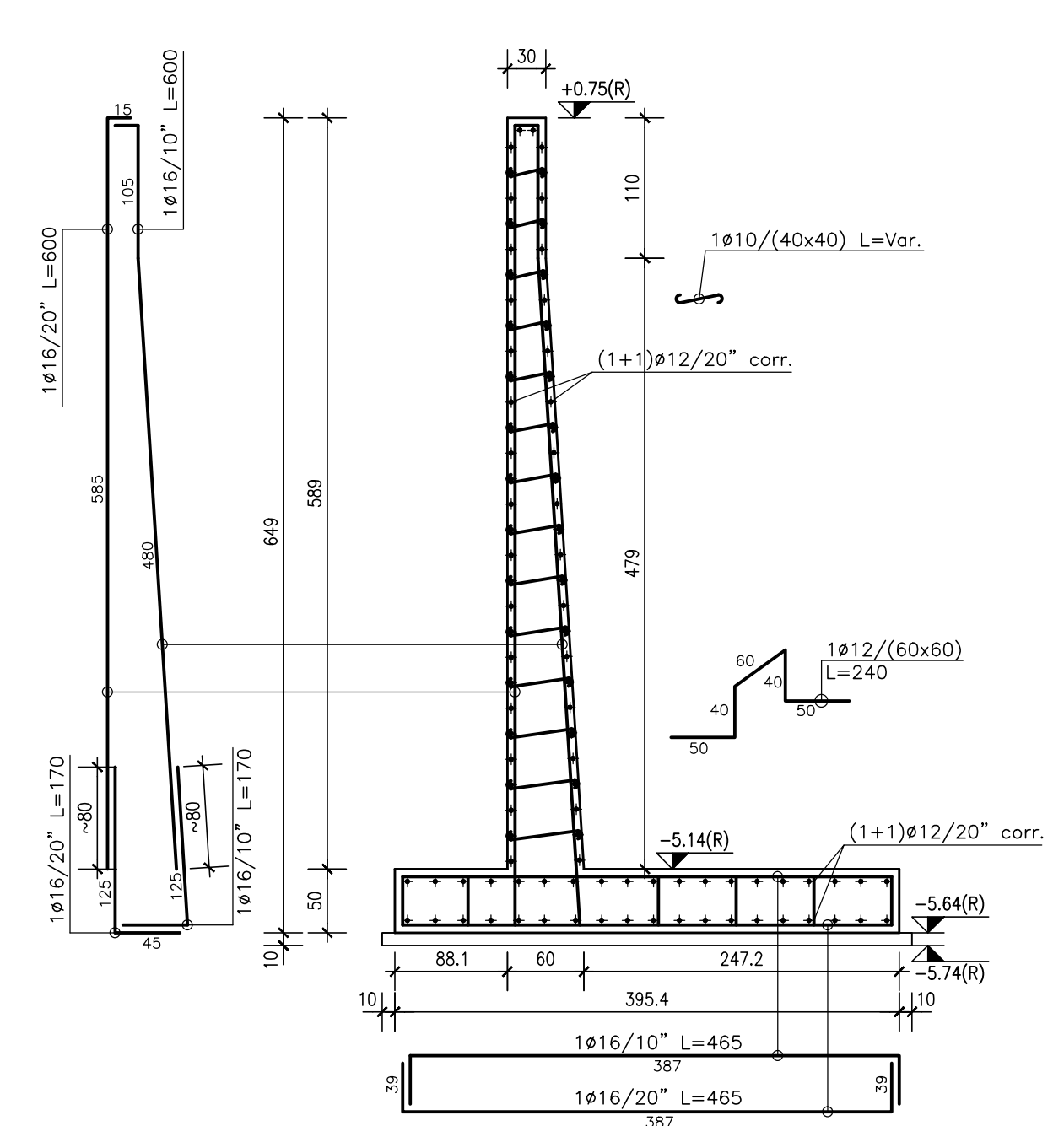
SEZIONE 1-1
